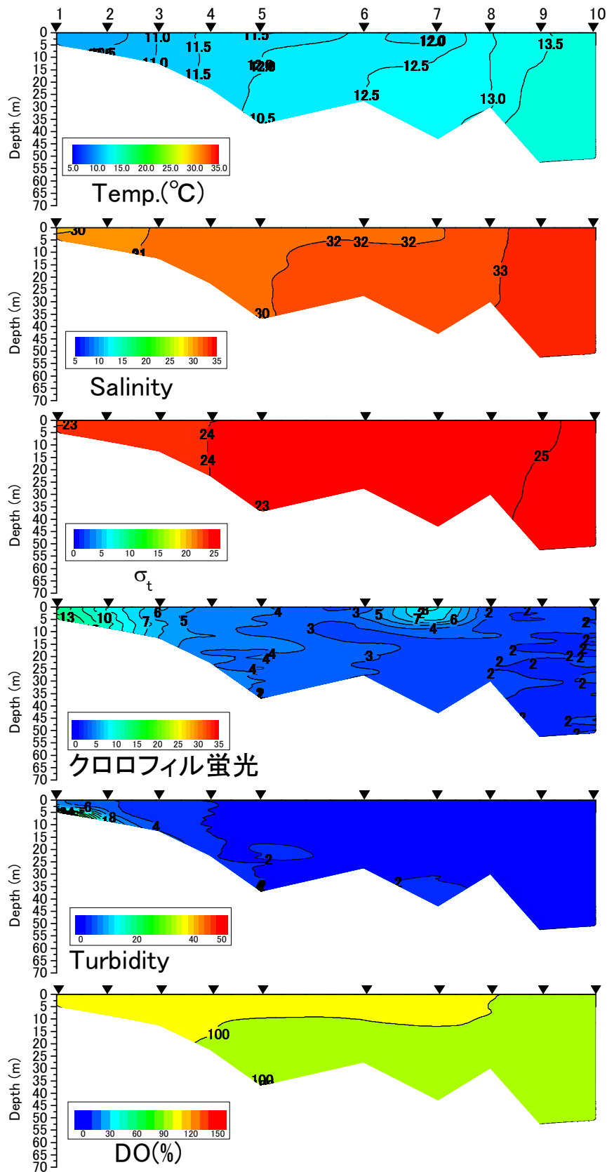
有明海中央ラインの水温(°C)、塩分、密度( \sigma_t )、クロロフィル蛍光強度、濁度、溶存酸素飽和度(DO%)の鉛直面図(国土交通省の調査による) (2017年2月1日)
